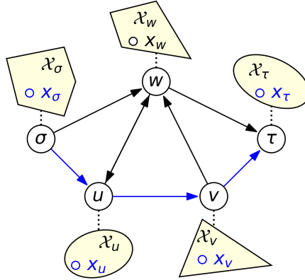
Hình 4.15: Minh họa bài toán SPP in GCS. Mỗi đỉnh i \in \{\sigma, u, v, w, \tau\} trong đồ thị được liên kết với một biến liên tục x_i nằm trong một tập lồi tương ứng \mathcal{X}_i . Trọng số của mỗi cạnh là một hàm lồi của các biến liên tục tại hai đỉnh mà cạnh đó kết nối. Trong hình, đường đi màu xanh p = (\sigma, u, v, \tau) thể hiện một nghiệm khả thi của thành phần rời rạc, trong đó tổng chi phí phụ thuộc vào các giá trị tối ưu của x_\sigma, x_u, x_v, x_\tau nhưng độc lập với x_w [16].
